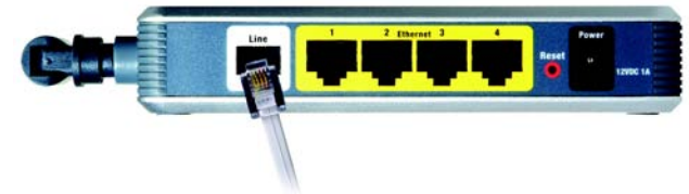
Abbildung 4-1: Herstellen der ADSL-Verbindung
